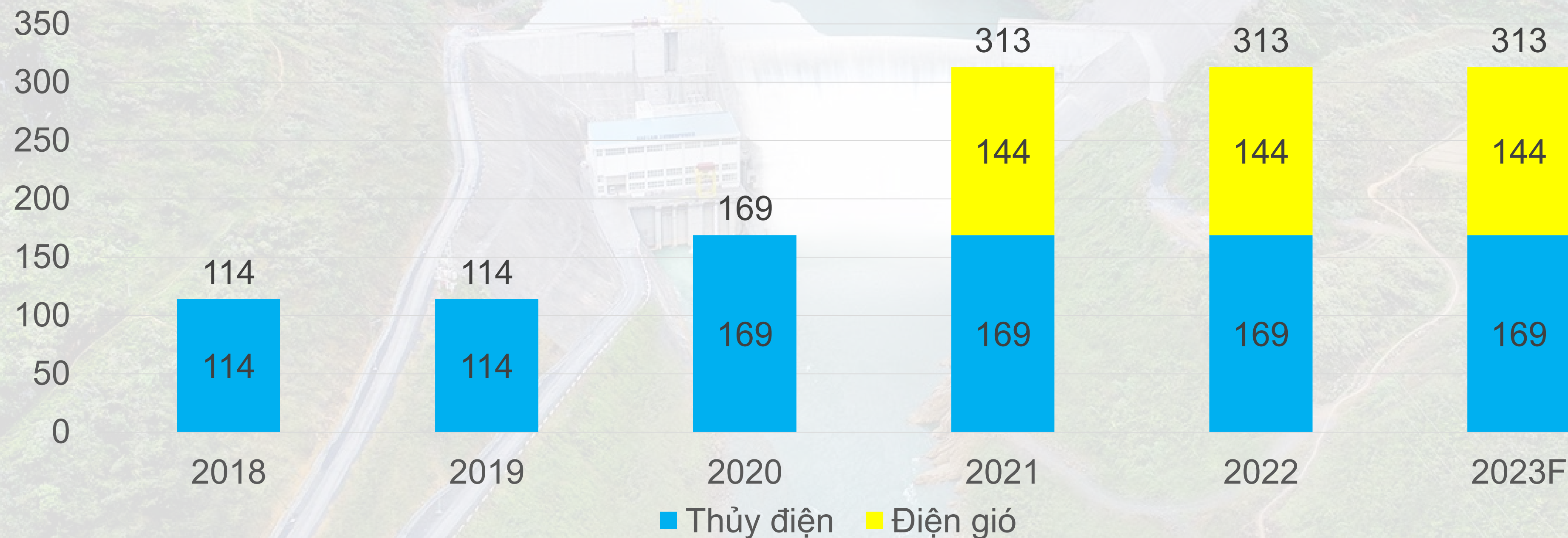
Lũy kế công suất theo thời điểm phát điện (MW)
